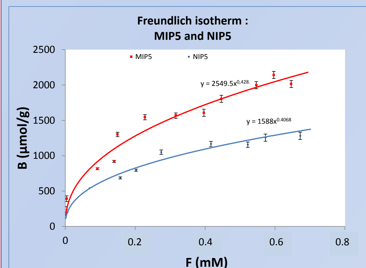
Fig. 2 : Freundlich isotherm example MIP5 and NIP5.
