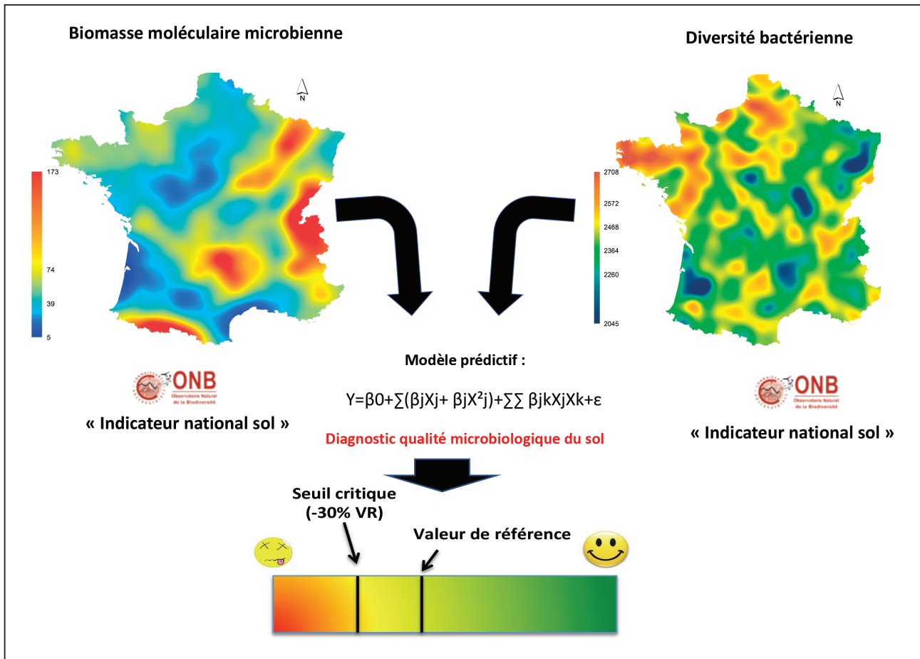
Figure 7 : Élaboration d'indicateurs microbiens de la qualité des sols à partir du RMQS.
