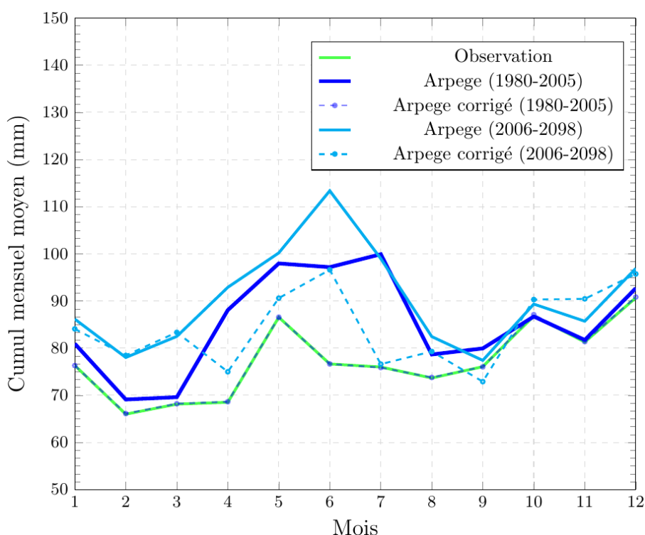
Figure 27 : a) Cycle annuel moyen des pluies non-corrigées et corrigées simulées par Arpege (CNRM-CM5.1) sur la Bourgogne pour la période historique (1980-2005) et projeté (2006-2098)
