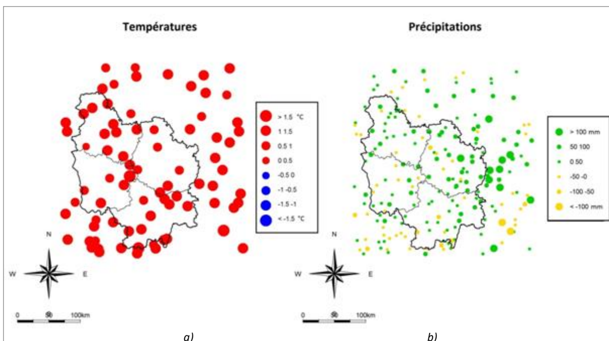
Figure 13 : Cartes des différences (période 1988-2011 moins période 1961-1988) des températures moyennes annuelles (a) et des cumuls annuels moyens (b) pour les stations de la région Bourgogne élargie
