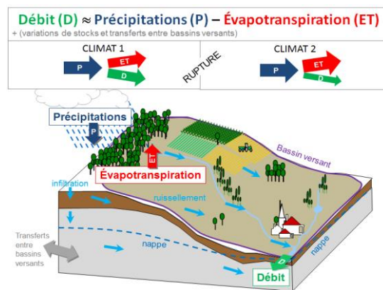
Figure 4 : Schéma simplifié du cycle de l'eau à l'échelle d'un bassin versant (d'après Ubertosì)
