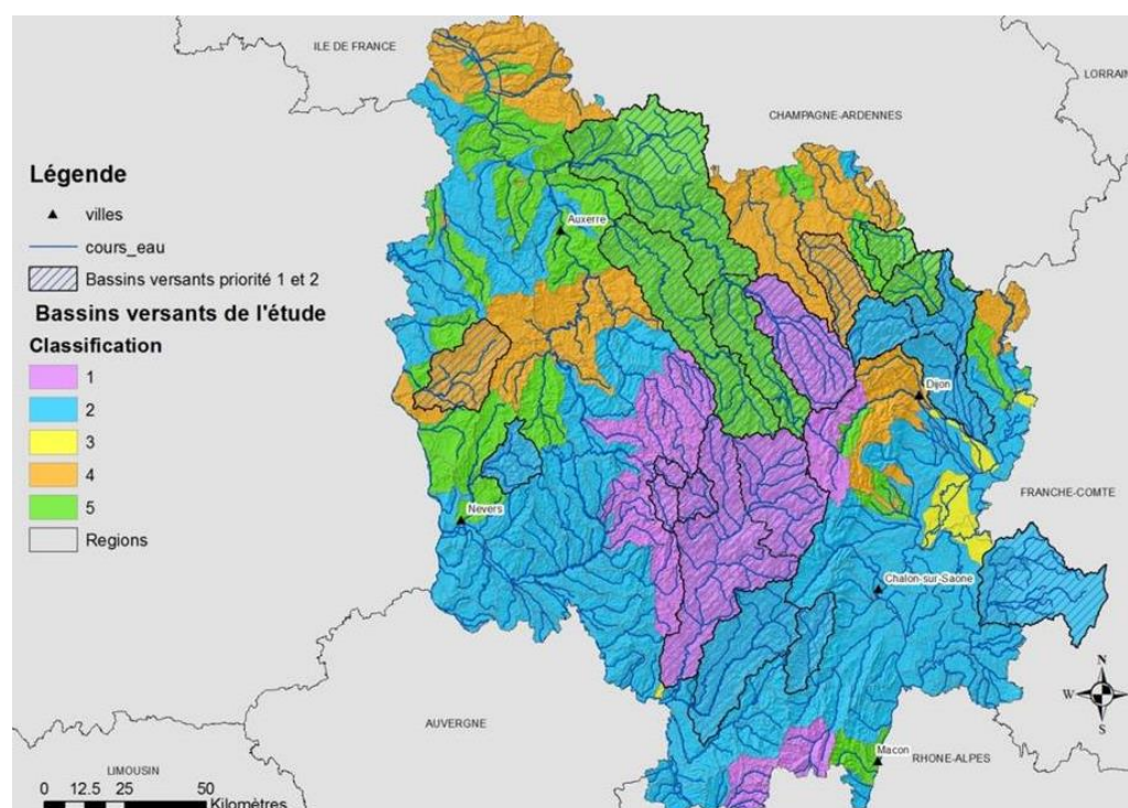
Figure 6 : Carte présentant les bassins versants selon la typologie du BRGM (5 grands types de fonctionnement hydrologique identifiés)
