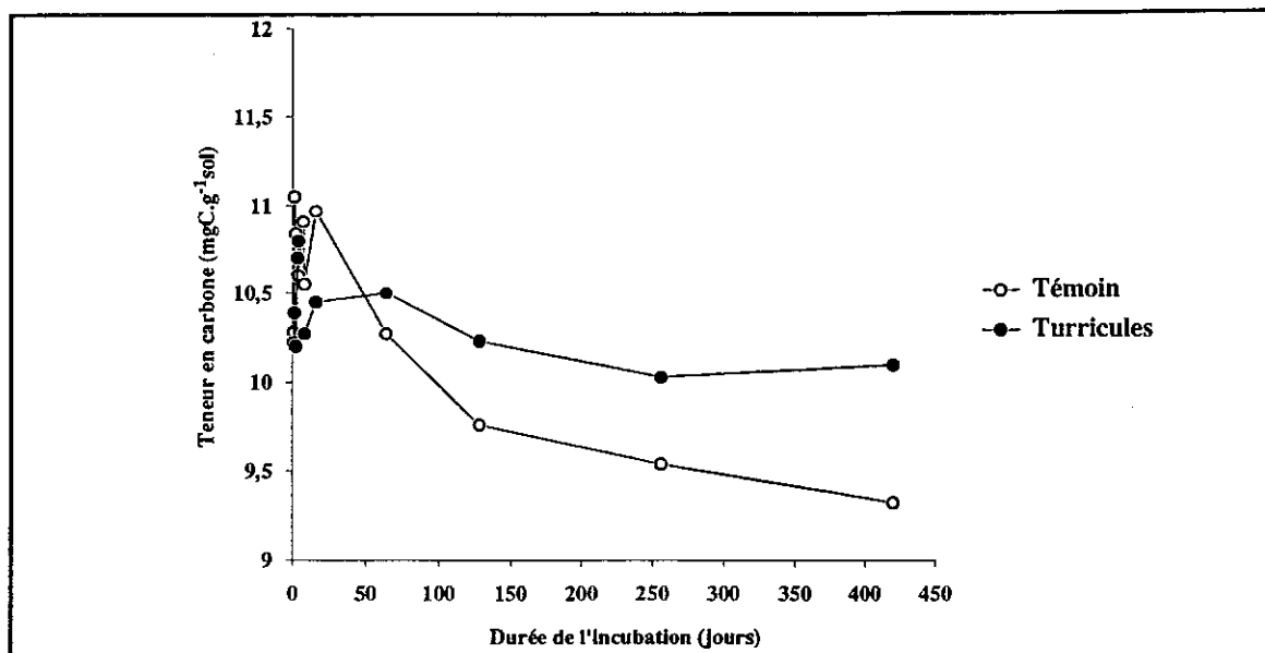
Figure 4 : Variations des teneurs en carbone ( \text{mg C.g}^{-1} \text{sol} ) d'un sol ferrugineux sableux (Lamto, Côte-d'Ivoire) au cours d'une incubation ( T = 28^\circ\text{C} , \text{H}_2\text{O} \% = 12 ) de longue durée, en relation avec l'activité de Millsonia anomala .
