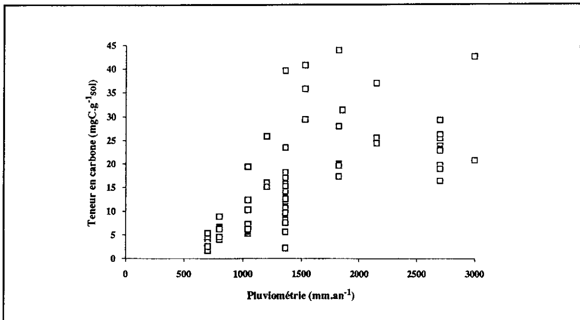
Figure 1 a : Relation teneur en carbone-pluviométrie moyenne annuelle. Horizons 0-10 cm. Situations d'Afrique de l'Ouest, des Petites Antilles et du Brésil.
